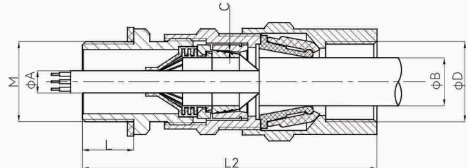
钢管布线
