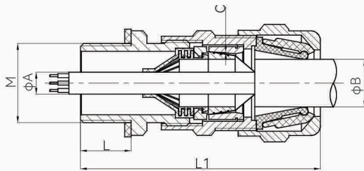
电缆布线
